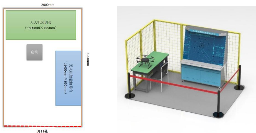
图 1 无人机装调检修赛位布局图
