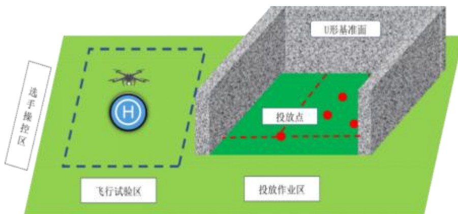
图 2 无人机测试及定点投放布局图
